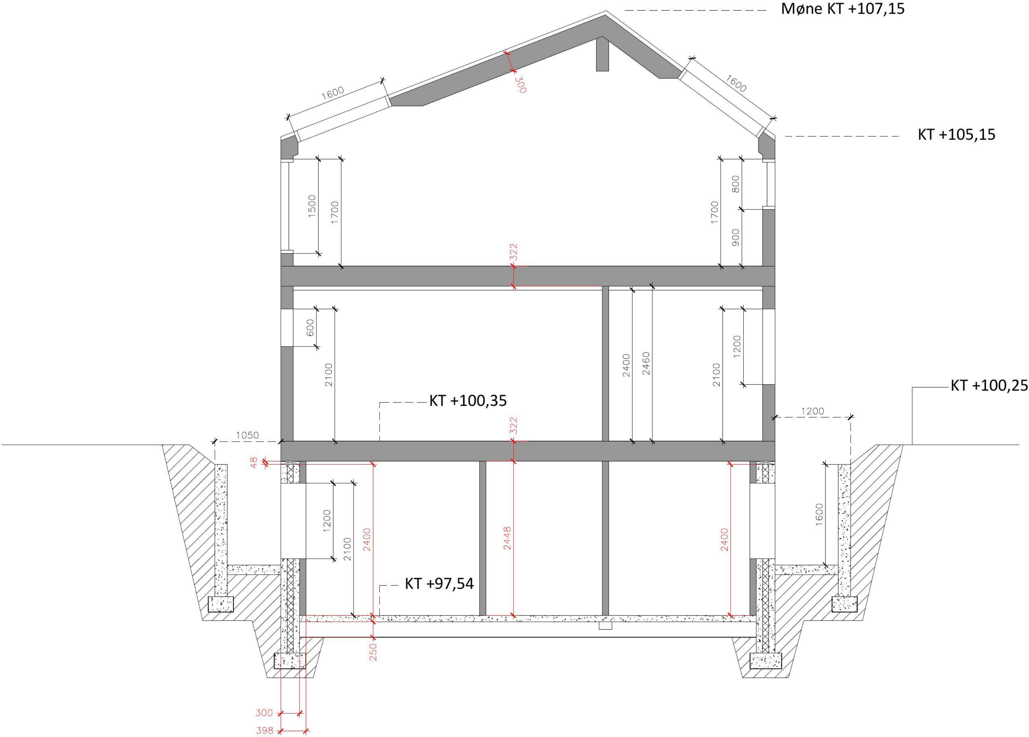
SNITT A:A
